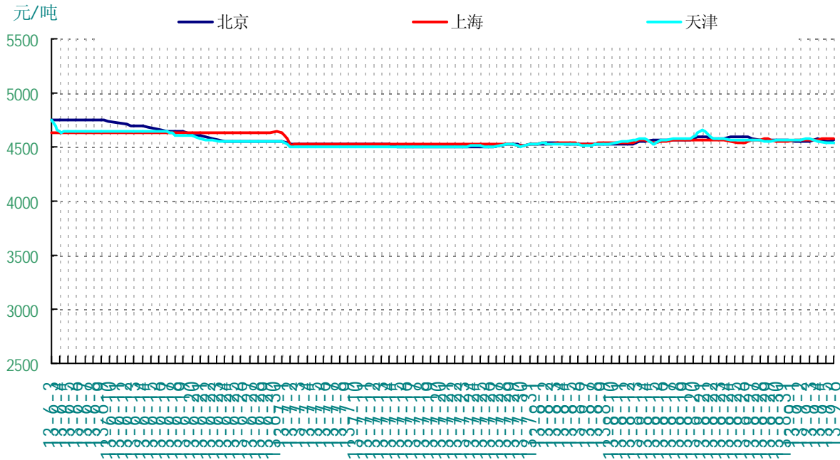
2013年6月至今重点城市冷板(1mm)日价格走势
