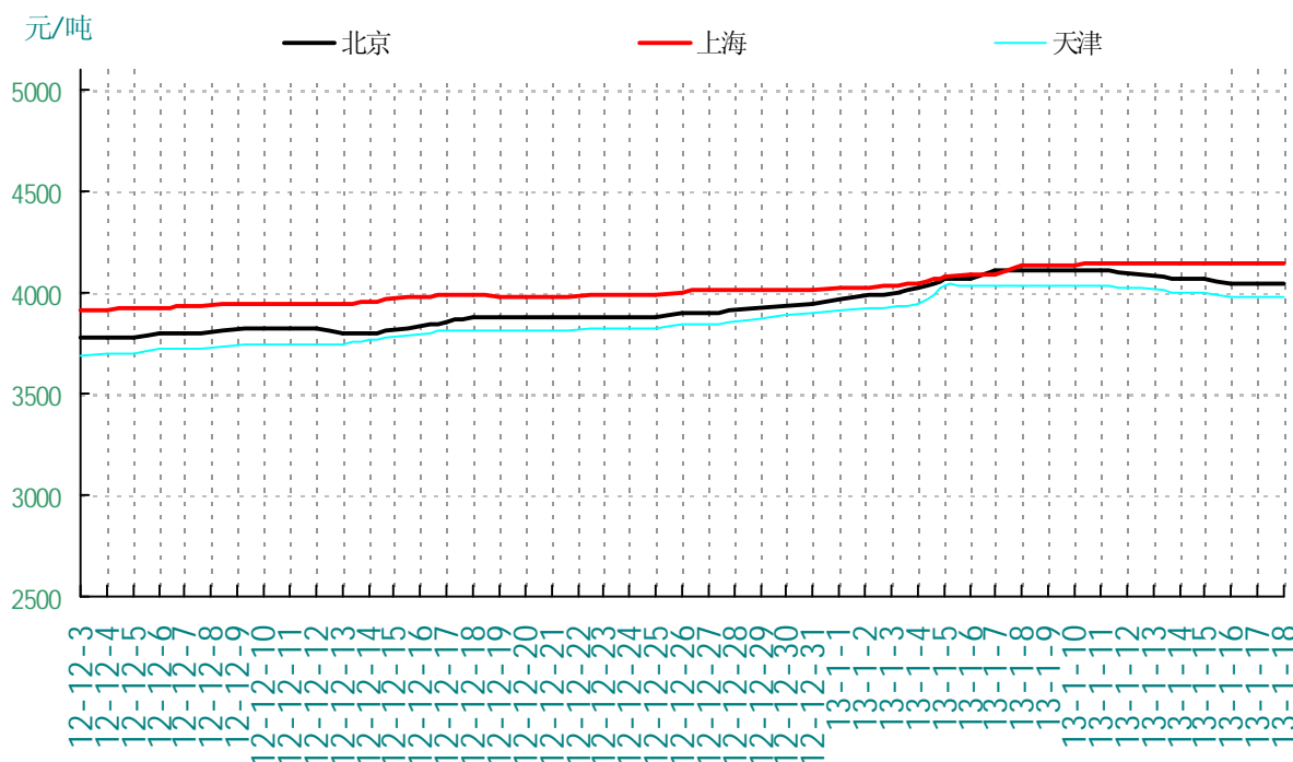
2012年12月至今重点城市热卷日价格走势
